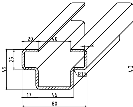
Standard profil guide weight: ca. 4,8 kg/m
